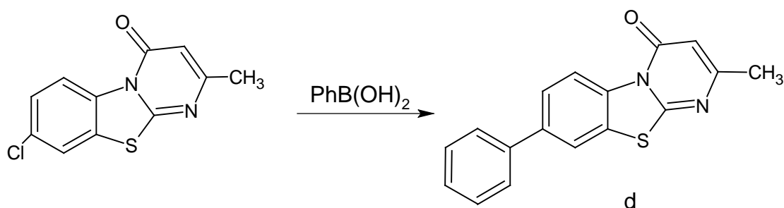
Схема 2. Синтез 8-фенил-2-метил-бензо[4,5][1,3]тиазоло[3,2-а]пиримидин
