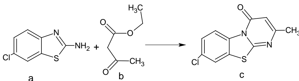
Схема 1. Синтез 8-хлор-2-метил-бензо[4,5][1,3]тиазоло[3,2-а]пиримидин.
