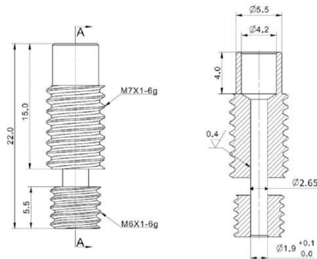
Рис.1 Биметаллический термобарьер.
