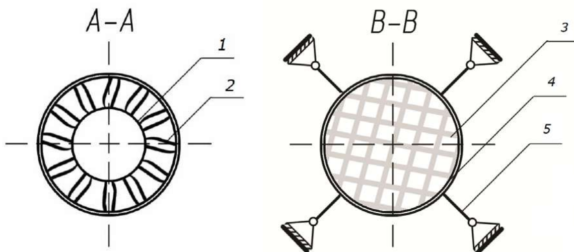
Рисунок 1. Дополнительное средство эвакуации с верхних этажей МЦК в разрезе: 1 – тормозное средство 2 – гибкие связи тормозного устройства 3 – эластическая сетка 4 и 5 – кольцо с растяжками.
