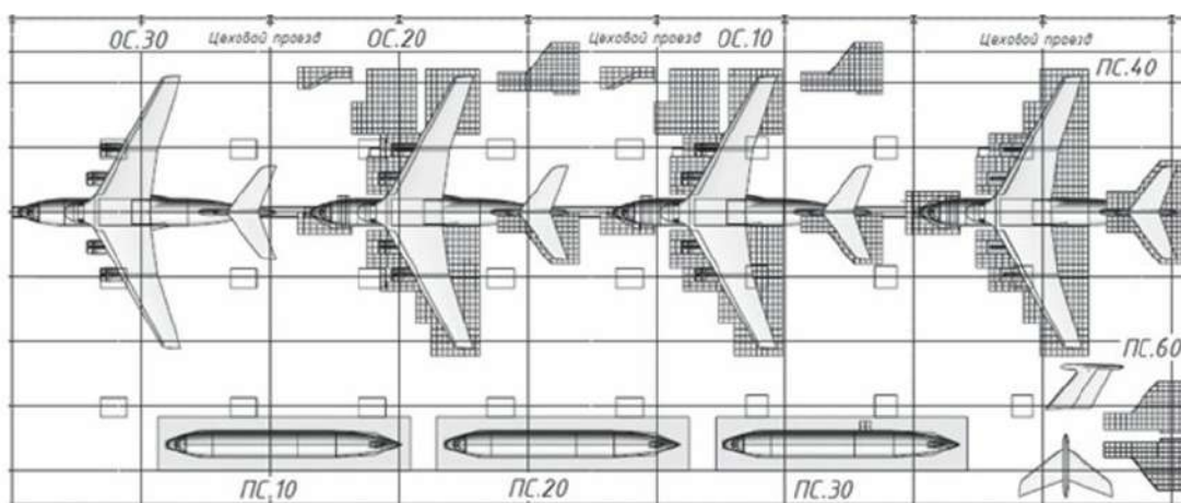
Рис. 1. Схема ПЛС.
