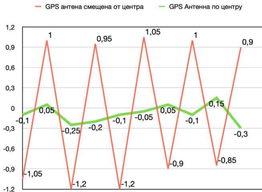
Рис. 5. График сравнения ошибок измерений точности.
