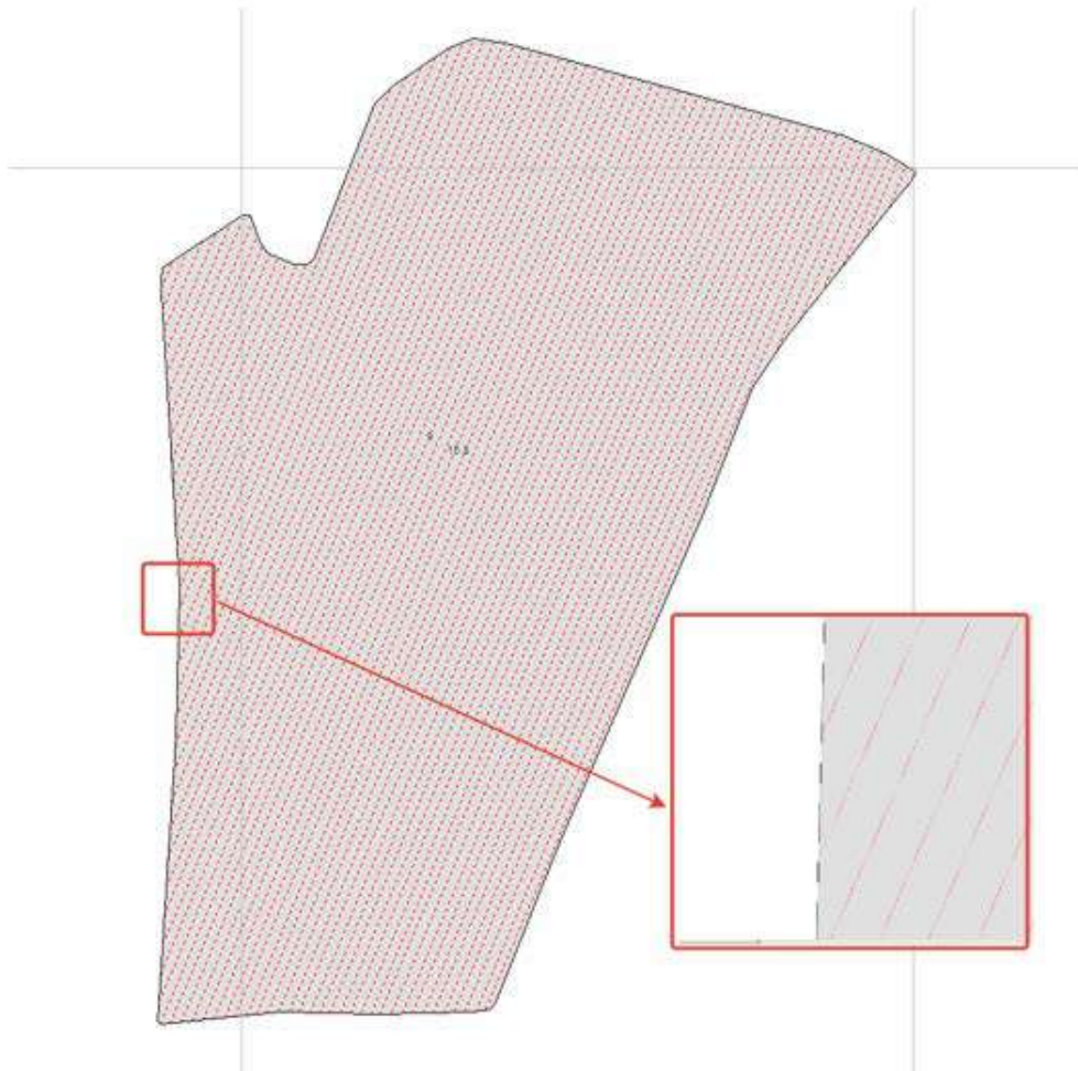
Рис. 4. Картографическая схема траекторий обработки.
