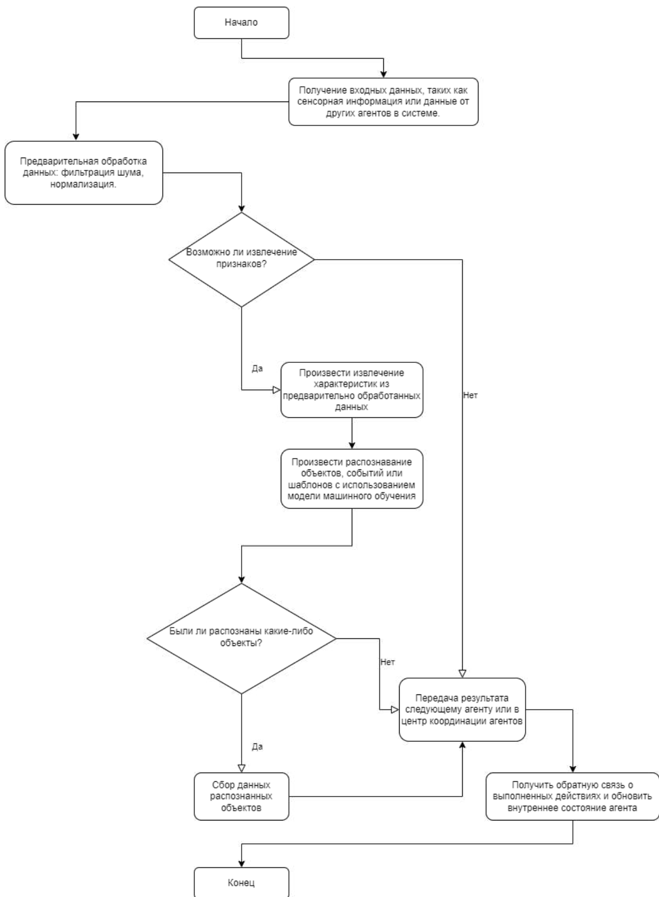
Рис. 1. Алгоритм работы интеллектуального агента распознавания
