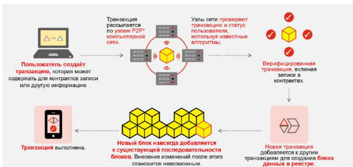
Рис. 1. Функциональная схема работы блокчейн-технологии
