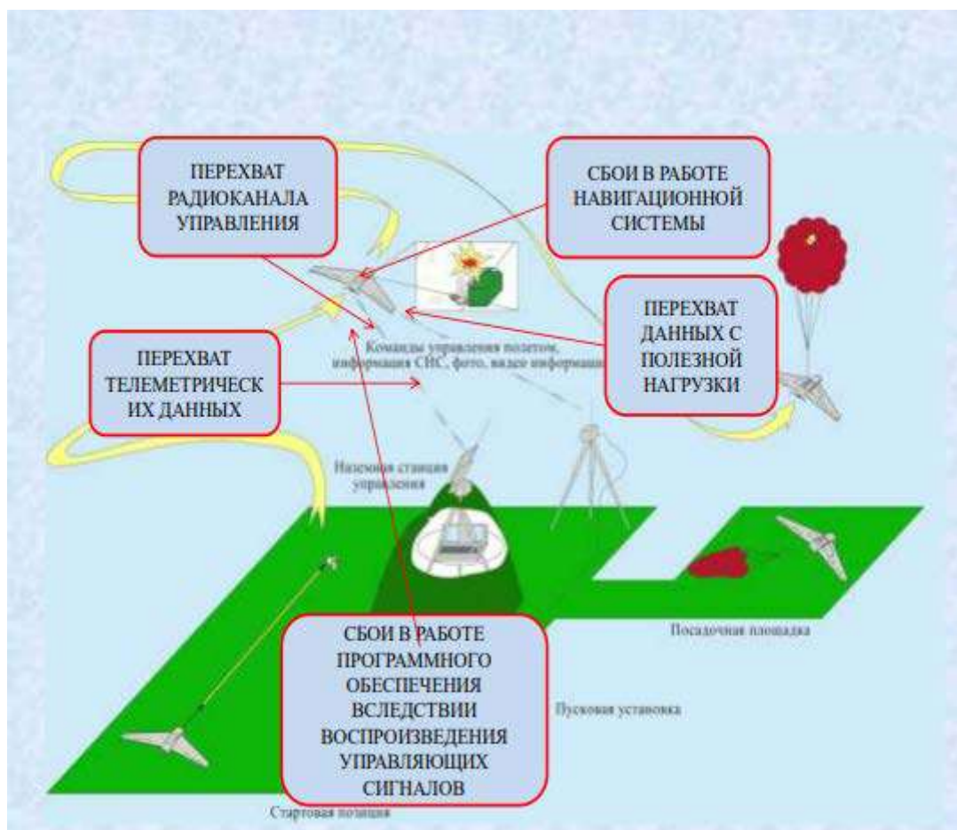
Рисунок 1. Уязвимости в контурах управления БПЛА ближнего действия.
